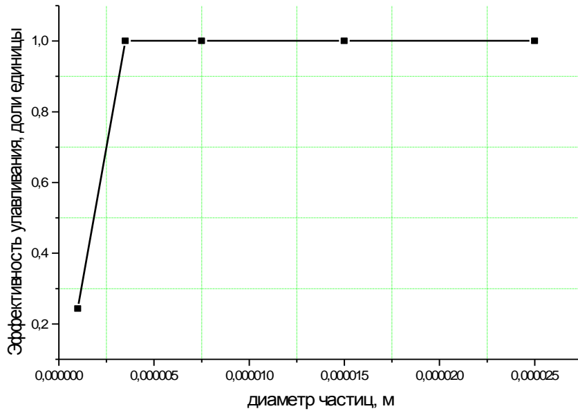
Зависимость эффективности улавливания от диаметра частиц пыли
