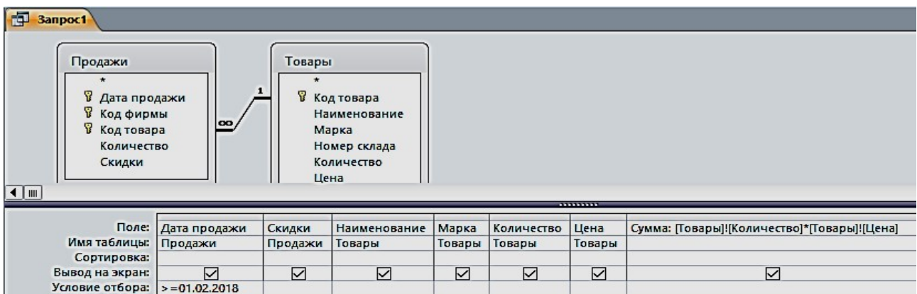
Рис. 3.8. Запрос «Стоимость» в режиме Конструктора
