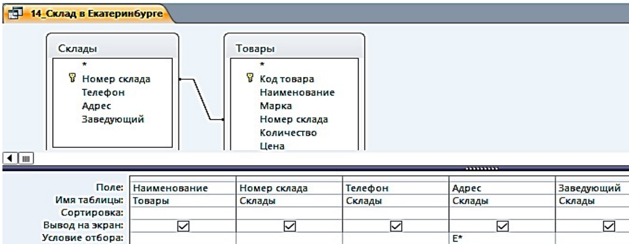
Рис. 3.6. Запрос «Склад в Екатеринбурге» в режиме Конструктора
