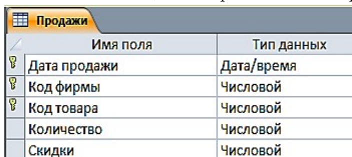
Рис. 1.13. Окно таблицы «Продажи» в режиме «Конструктора»
